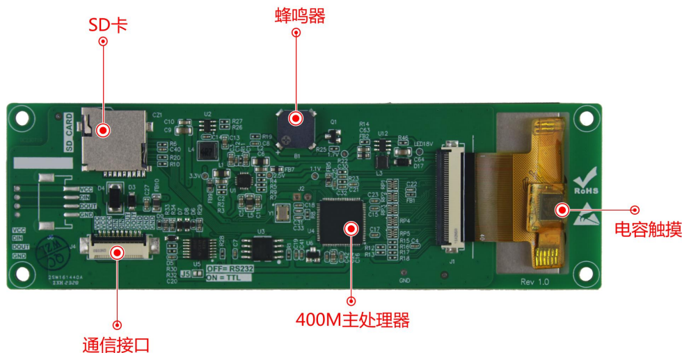
图 1-3 硬件配置图
