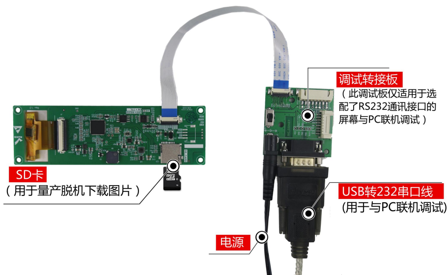
图 1-4 调试工具图
